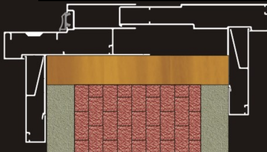
Ugradnja u zid 130mm sa drvenim slepim ramom
