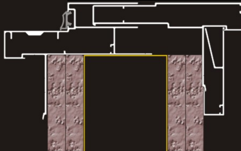
Ugradnja u zid 130mm sa drvenim slepim ramom
