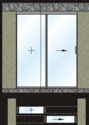
Jednokrilno klizno i fiksno
