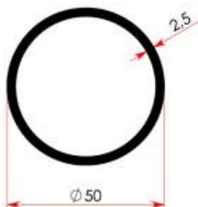
MK02A 1,011 kg/m
