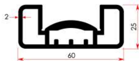
MK31 1,265 kg/m
