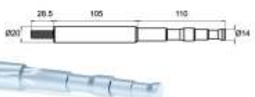
Anker 105 mm sa navojem za stub Ø 40
