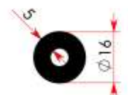
MK41B 0,470 kg/m
