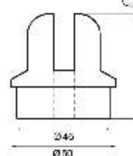
Ø 50 Deo zglobnog držača A
