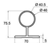
Držač za zid rukohvata Ø40 - prsten
