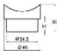
Ø 40 Veza na Ø 40 rukohvat
