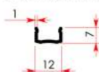
6969 0,065 kg/m
