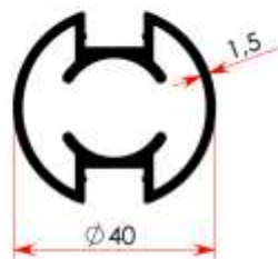
6360 0,780 kg/m
