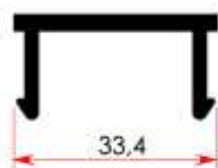
MK32 0,120 kg/m
