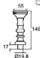
Ø 40 Dekorativni zglobni držač
