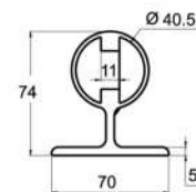
Držač za zid stuba Ø 40 - prsten
