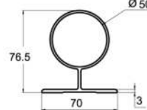
Držač za zid rukohvata Ø50 - prsten
