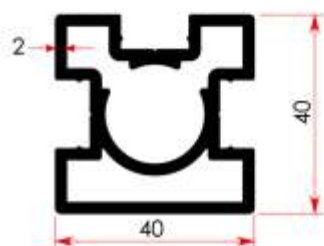
MK33 1,274 kg/m
