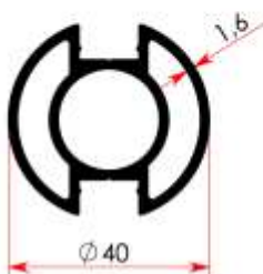
7178 0,895 kg/m
