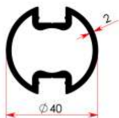
MK20D 0,840 kg/m
