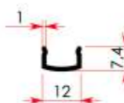
MK50K 0,065 kg/m
