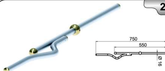
Ukrasni element Ø 16 C
