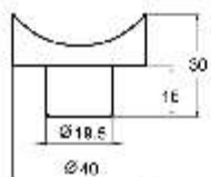
Ø 40 Veza stub na Ø 50 rukohvat
