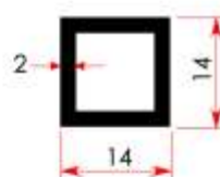
MK37 0,260 kg/m
