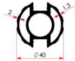
6968 0,979 kg/m
