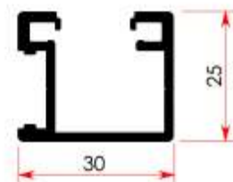
MK35 0,550 kg/m
